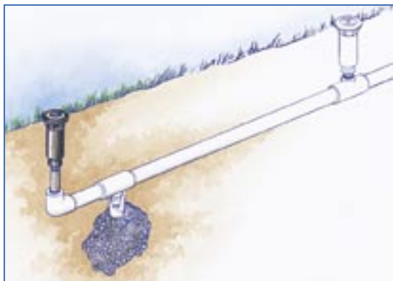
Instalación de la Válvula de Drenaje Automática para los Climas con Temperaturas Bajo Cero: Coloque las válvulas de drenaje en los lugares más bajos en cada una de las zonas.
